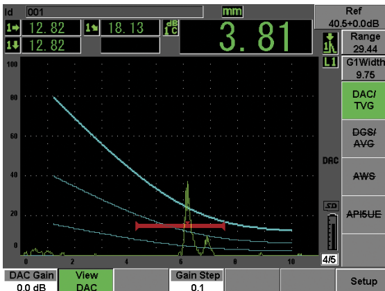
EPOCH 600型仪器的动态DAC/TVG特性
