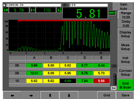
EPOCH 600型仪器的腐蚀模块特性
