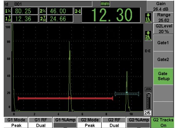
EPOCH 600型仪器的回波到回波性能，带有闸门跟踪。
