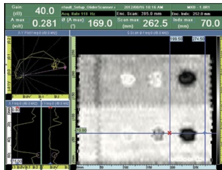
Высокочастотное сканирование; фазовый С-скан, отличная цветовая палитра
