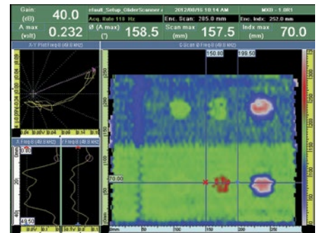
Высокочастотное сканирование; фазовый С-скан, курсор над расслоением
