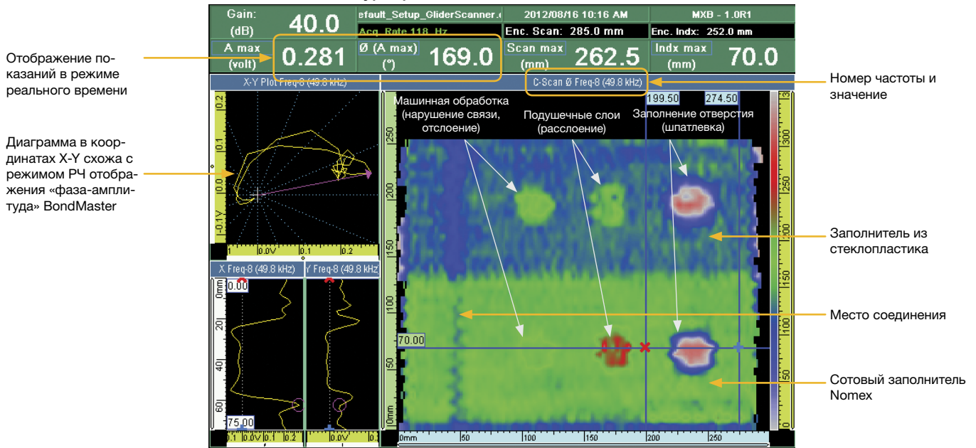
Фазовый С-скан, курсор на заливке
