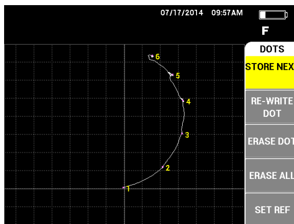
Le système de points de référence amélioré du BondMaster 600.
