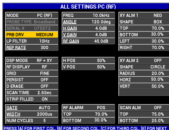
Écran permettant de modifier rapidement tous les paramètres.
