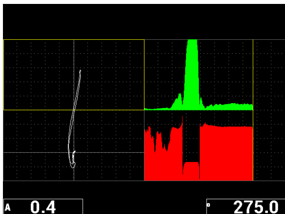
Mode MIA muni d'une nouvelle vue de balayage et de lectures en temps réel.
