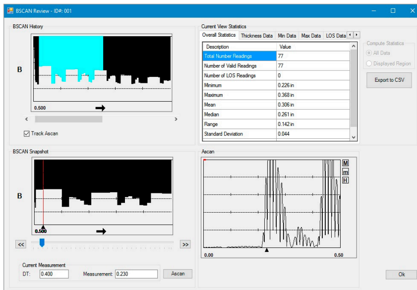
GageView的Thickness（厚度）程序中的B扫描查看功能
