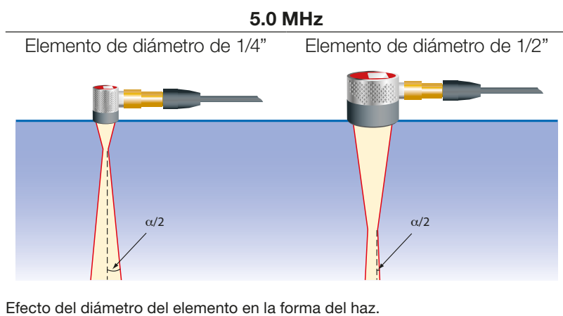
Efecto del diámetro del elemento en la forma del haz.
