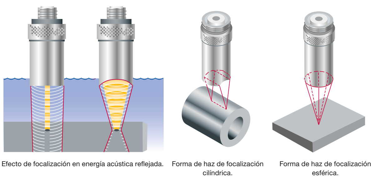
Efecto de focalización en energía acústica reflejada. Forma de haz de focalización cilíndrica. Forma de haz de focalización esférica.
