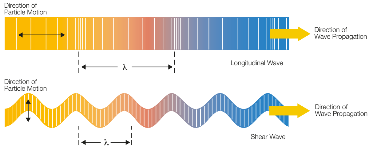
Comparación del movimiento de partículas en los modos de onda longitudinal y transversal.
